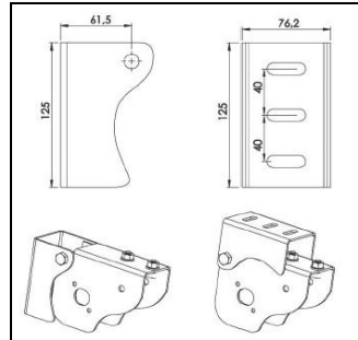
МОНТАЖНИ КОНЗОЛИ
