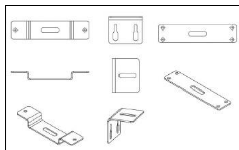
МОНТАЖНИ КОНЗОЛИ
