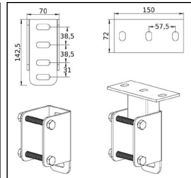
МОНТАЖНИ КОНЗОЛИ
