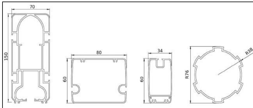
ПРОФИЛИ
