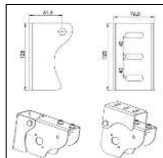
МОНТАЖНИ КОНЗОЛИ
